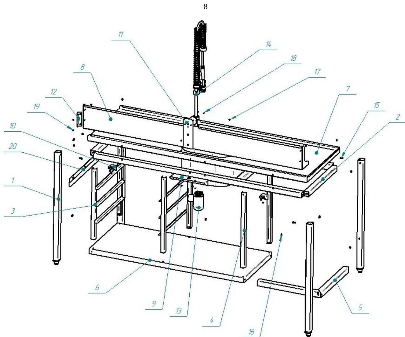
Рис.2 Схема сборки стола предмоечного СПМП-7-7
