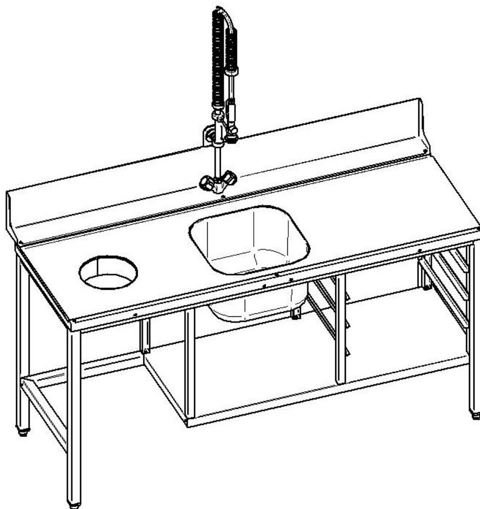
Рис.1 Стол предмоечный СПМП-7-7
